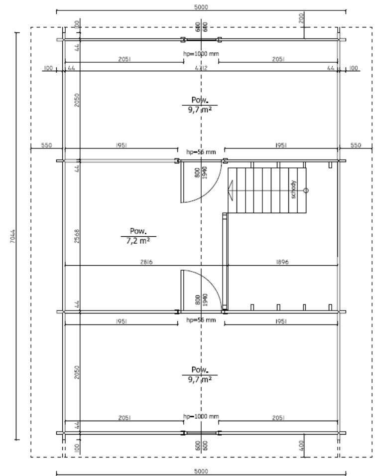
RZUT PODDASZA
