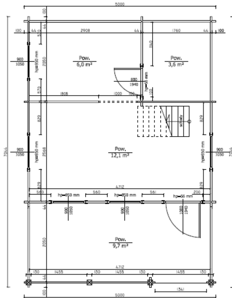
RZUT PRZYZIEMIA
